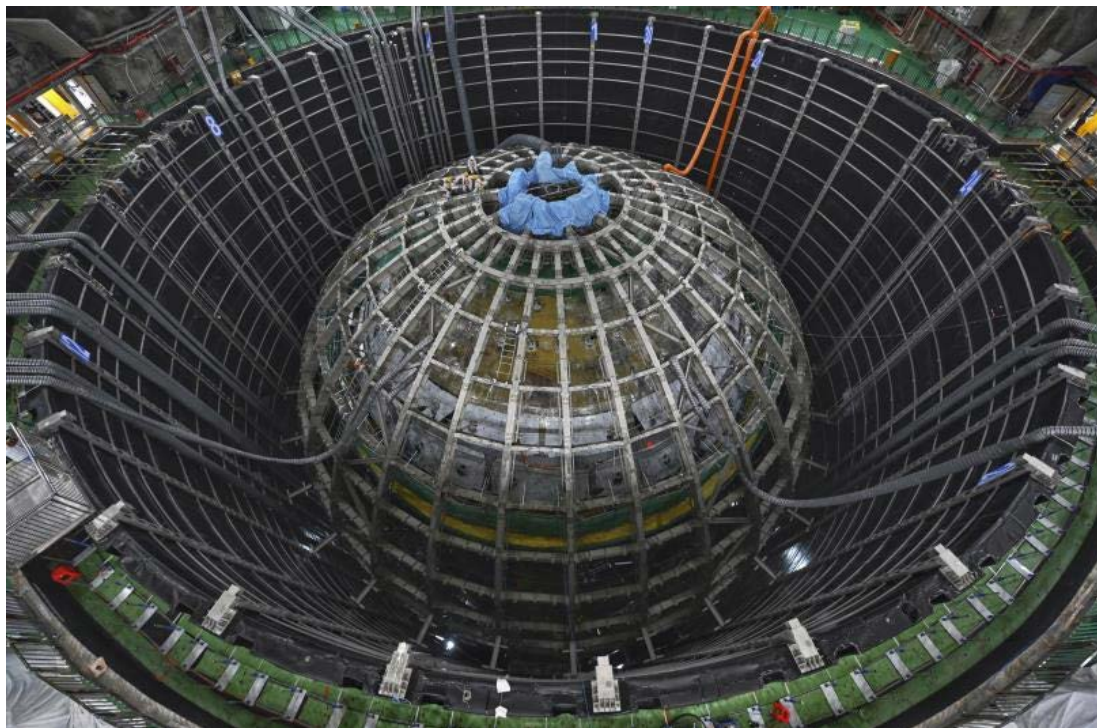
Рис. 16. Текущее состояние сборки детектора JUNO
