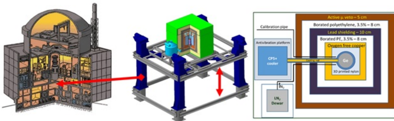
Рис. 18. Схема установки vGeN, нацеленной на детектирование CEvNS. Установка расположена непосредственно под реактором #3 КАЭС (слева), на специальном подъемном устройстве (в центре), позволяющем изменять поток антинейтрино в HPGe-детекторе, окруженном комплексной активной и пассивной защитой (справа)
